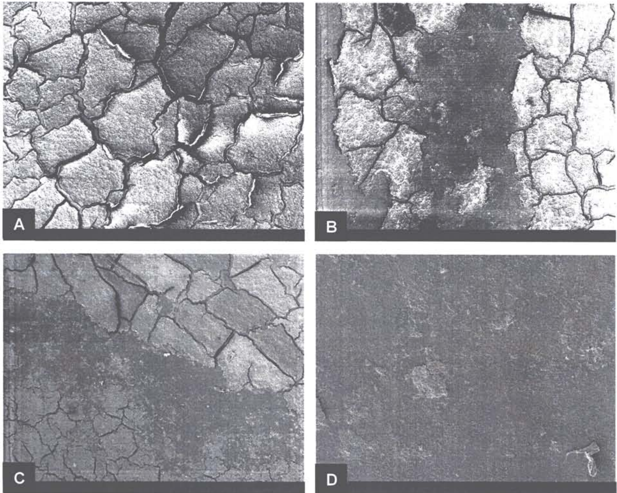
Abb. 3: REM-Aufnahmen der Oberfläche eines Silikonschlauchs mit einem 2 Jahre alten Biofilmbewuchs ohne Behandlung (A), nach 1000 Impulsen bei 0,5 bar Wasser- und 2,0 bar Luftdruck (B), nach 1000 Impulsen bei 1,0 bar Wasser- und 3,0 bar Luftdruck (C) und nach 4500 Impulsen bei 2,0 bar Wasserdruck und 3,0 bar Luftdruck (D). 1000fache Vergrößerung.
