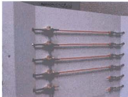
Abb. 1: Silikonschläuche mit Biofilm in der Versuchsanordnung zur Untersuchung des Impuls-Spül-Verfahrens
